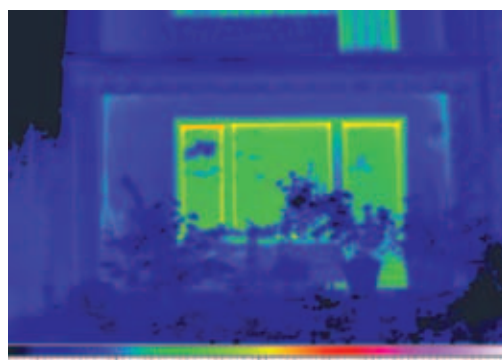
Na de zorgvuldige inbouw van Schüco Corona CT 70 ramen bewijst de thermografie het hoge energiegeïsoleerde nut van de investering. Het oorspronkelijke energieverlies wordt praktisch volledig vermeden.
