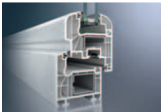
Schüco Corona CT 70 Rondo
