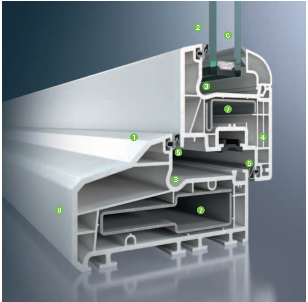
Schüco Corona CT 70 Accent
